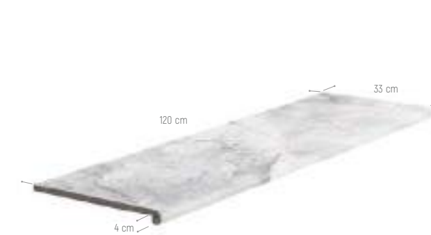
PELDAÑO ML 120 33 x 120 x 4 cm - 13.0"x 47.2"x 1.6" 13 mm rectificado, rectified C-1/C-3
