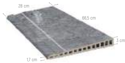
BORDE DESBORDANTE 28 x 66,5 cm - 11.0"x26.2" rectificado, rectified C-3
